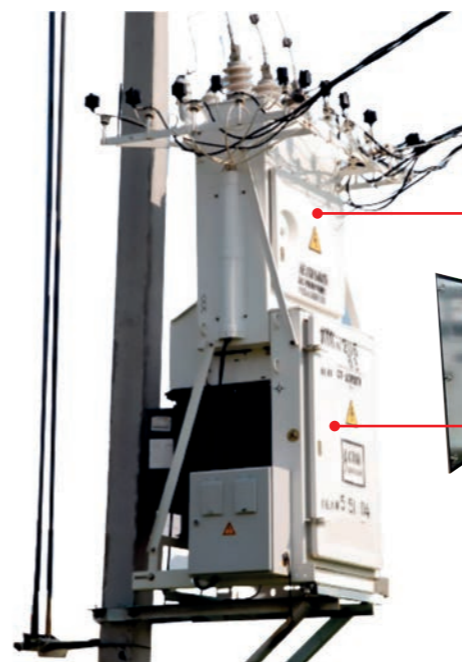
ПОДСТАНЦИИ ТРАНСФОРМАТОРНЫЕ МАЧТОВЫЕ ТИПА МТП мощностью от 25 до 100 кВ*А напряжением 6 (10) кВ
