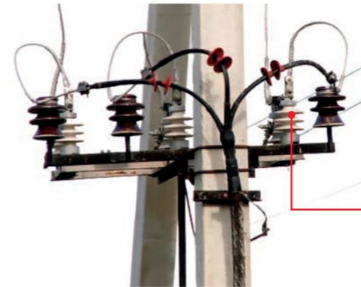
РАЗЪЕДИНИТЕЛИ ПЕРЕМЕННОГО ТОКА НА НАПРЯЖЕНИЕ 10кВ НАРУЖНОЙ УСТАНОВКИ РЛНГ-3-2-10/400 У1
