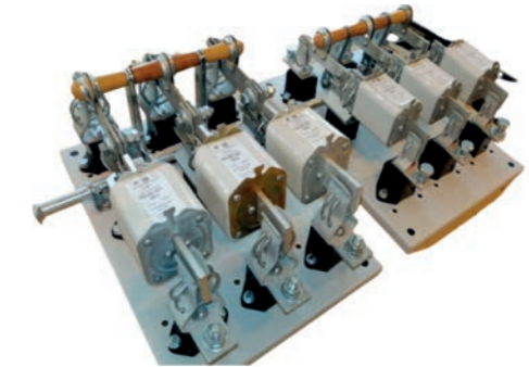
ВЫКЛЮЧАТЕЛИ-РАЗЪЕДИНИТЕЛИ НИЗКОВОЛЬТНЫЕ на номинальные токи 100, 250 и 400А
