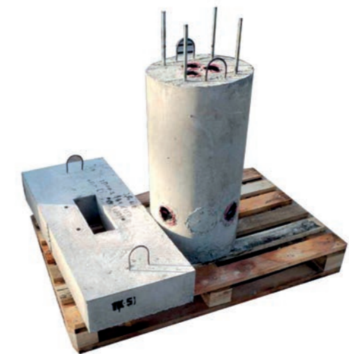
Фундаменты для станций зарядки автомобилей и ВРУ
