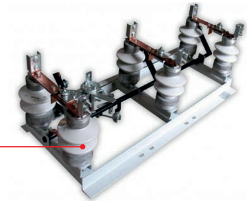
РАЗЪЕДИНИТЕЛИ ПЕРЕМЕННОГО ТОКА НА НАПРЯЖЕНИЕ 10кВ НАРУЖНОЙ УСТАНОВКИ РЛНГ-3-2-10/400 У1
