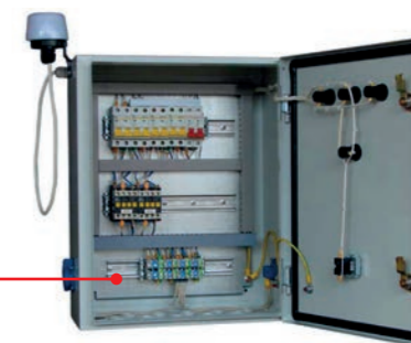
ШКАФ УПРАВЛЕНИЯ НАРУЖНЫМ ОСВЕЩЕНИЕМ ШУНО
